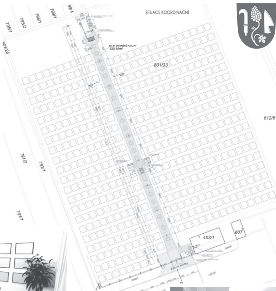
Situční výkres rekonstrukce přístupového chodníku.
